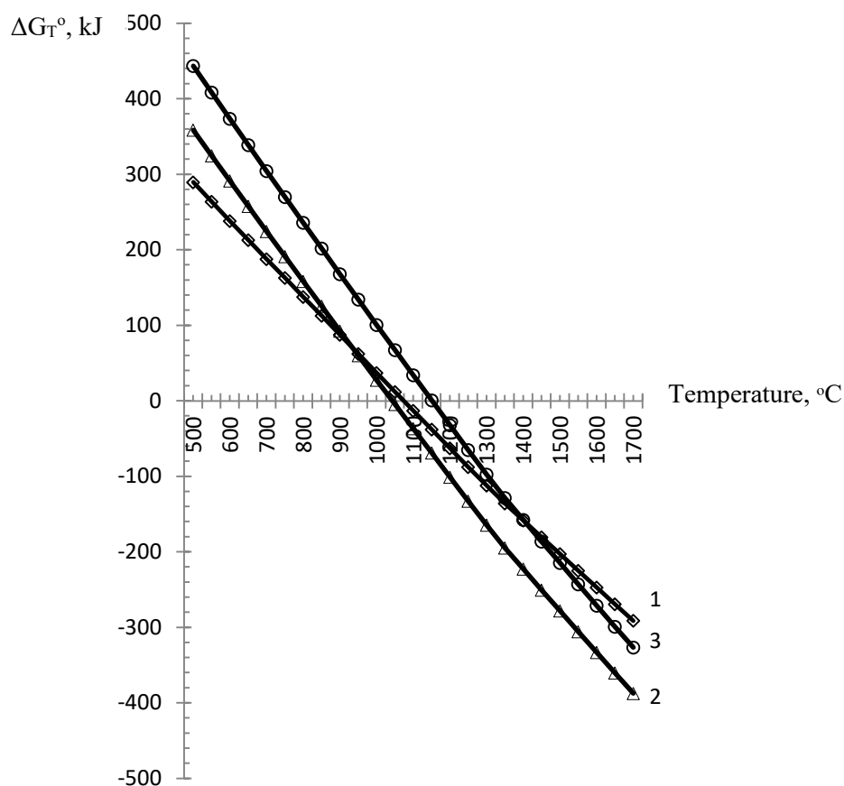
1- \text{ZnO} + 2\text{CaCO}_3 + \text{SiO}_2 = \text{Zn} + \text{Ca}_2\text{SiO}_4 + 2\text{CO}_2 + 0,5\text{O}_2 ; 2- \text{ZnO} + 3\text{CaCO}_3 + \text{SiO}_2 = \text{Zn} + \text{Ca}_3\text{SiO}_5 + 3\text{CO}_2 + 0,5\text{O}_2 ; 3- \text{ZnO} + 3\text{CaCO}_3 + \text{Al}_2\text{O}_3 = \text{Zn} + \text{Ca}_3\text{Al}_2\text{O}_6 + 3\text{CO}_2 + 0,5\text{O}_2 .
